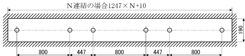
連結取付
