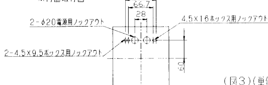
(図3)(単位:mm)
