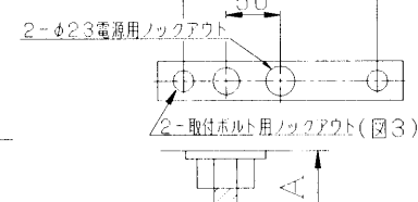
ボルト器具内寸法(図4)
