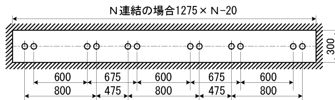
連結取付 (単体用器具の場合)
