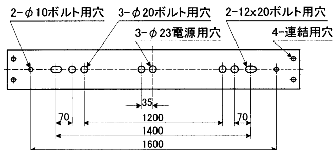
背面仕様図
