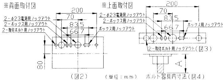
(図2) (単位: mm) ボルト器具内寸法(図4)
