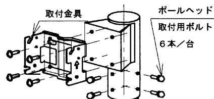
（図6A） 適合ポール：φ76.3
