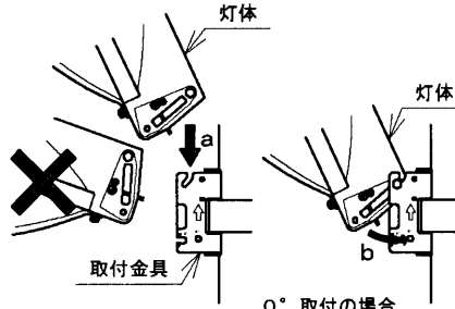
ボルト 灯体に仮組み品 外してください。 （図8）
