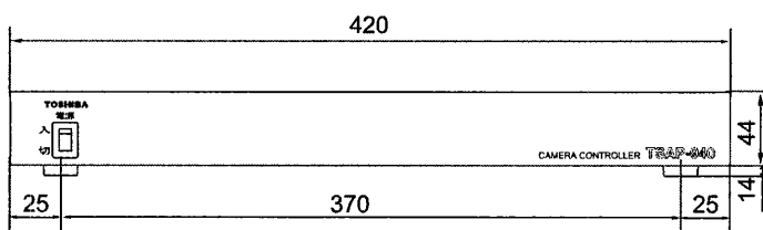
〔正面図〕
