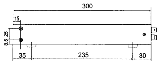
〔側面図〕
