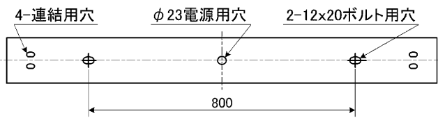
背面仕様図
