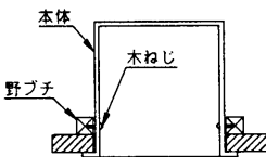
木ねじによる固定
