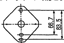
図4 サポート取付ピッチ
