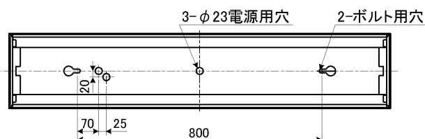
背面仕様図
