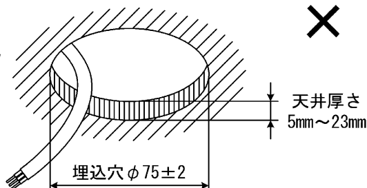
埋込穴寸法
