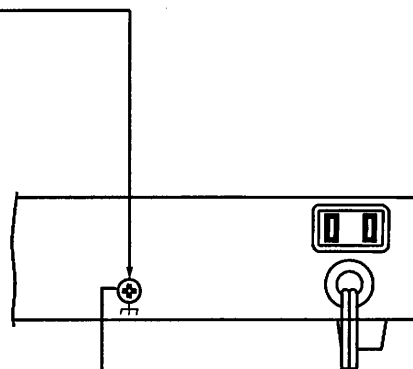
D種(第3種)接地工事
