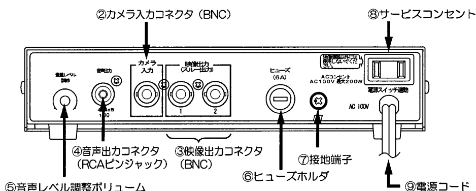
〔背面図〕
