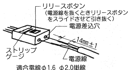
図－１ S L 端子台
