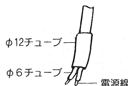
図－２ 保護チューブの取付方
