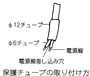
図-1 SL端子台
