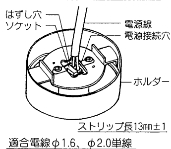
図－１ 電源線接続方法
