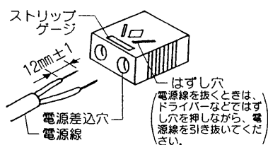
適合電線φ1.6、φ2.0単線 図-1 S L 端子台
