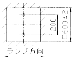
FHR-53310-PN9, 53311-PN9 FHR-54310-PN9, 54311-PN9 器具取付ボルトの寸法 器具内寸法 (A寸法) 60 mm
