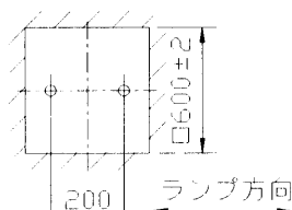
FHR-54300-PN9, 54301-PN9 器具取付ボルトの寸法 器具内寸法 (A寸法) 50 mm
