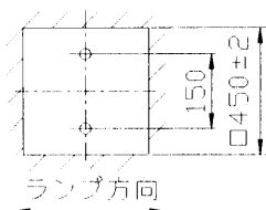
FHR-33321-PR9 器具取付ボルトの寸法 器具内寸法 (A寸法) 30 mm
