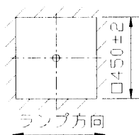
FHR-34321-PR9 器具取付ボルトの寸法 器具内寸法 (A寸法) 40 mm
