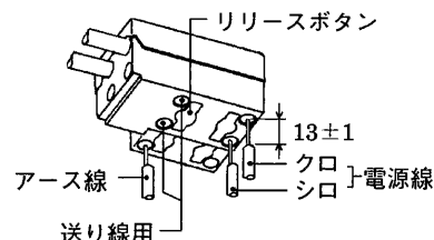
(適合電線 Ø1.6, Ø2.0 単線) 第2図
