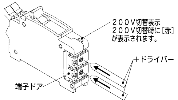
L1-L2 200V
