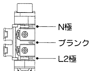
L2-N 100V
