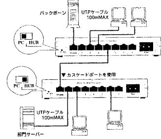
図4 カスケード接続の例(本製品同士)
