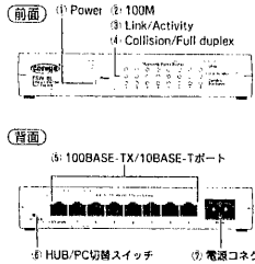
図1 外観図
