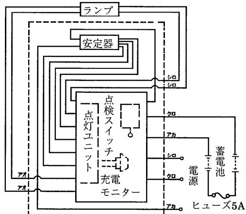
器具の回路図
