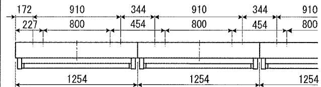
連結寸法図
