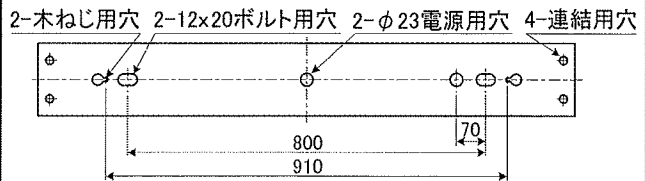
背面仕様図
