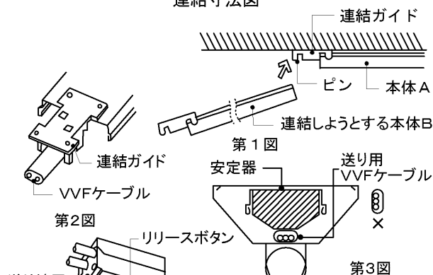
連結寸法図
