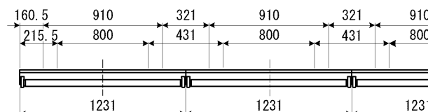
連結寸法図
