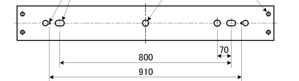
背面仕様図
