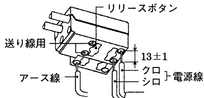
電源端子台
