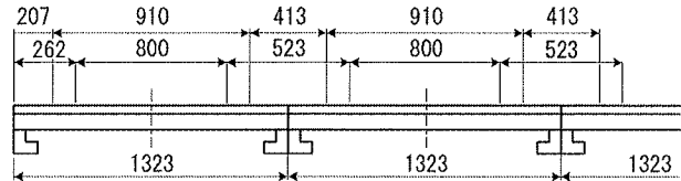
連結寸法図
