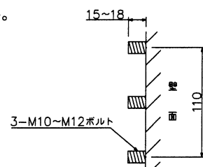
(図-1) 取付ボルト寸法
