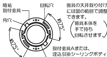
図-1 器具取付位置の調整
