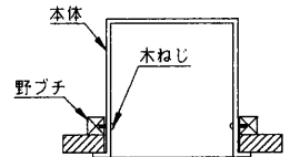
木ねじによる固定
