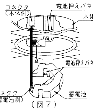
コネクタ(蓄電池側)
