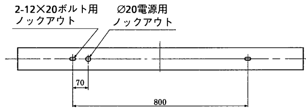
背面仕様図
