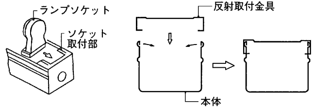
背面仕様図
