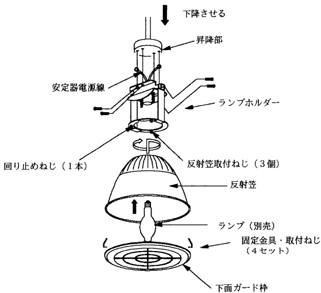
※図は安定器ボックスを取付けた場合の参考図です。
