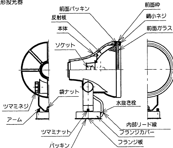
丸形投光器
