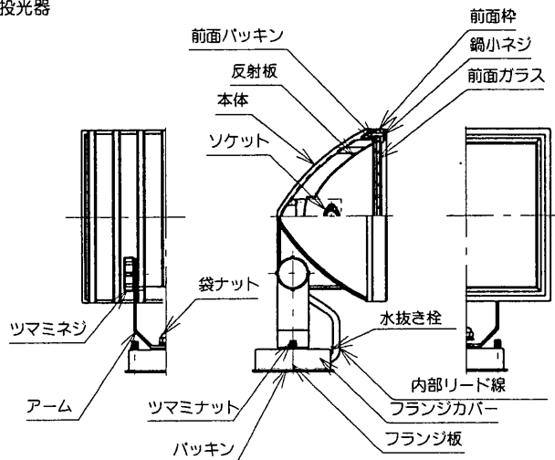
角形投光器
