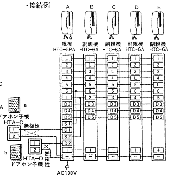
・接続例
