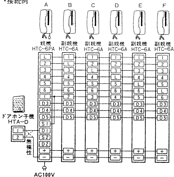
・接続例
