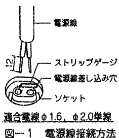
図-1 電源線接続方法
