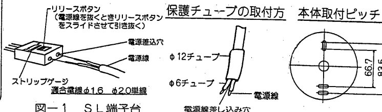
図-1 SL端子台
