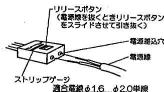
図-1 SL端子台
