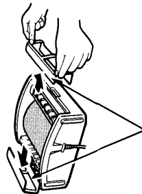
対向電極板 (2カ所)
