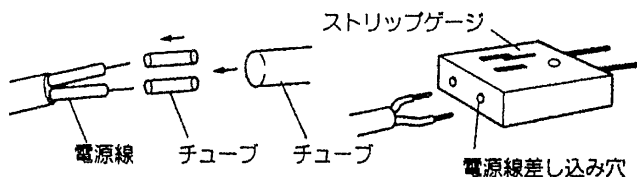
図 2 SL 端子台
