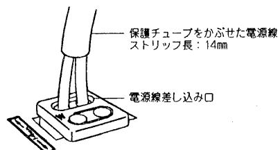
図-1 電源線接続方法
