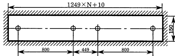
連結取付
