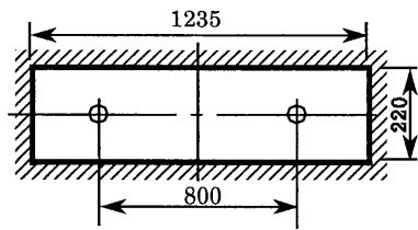
単体取付
