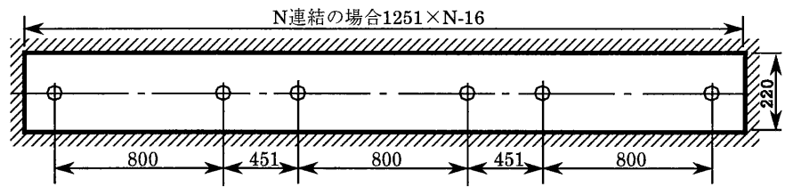
連結取付
