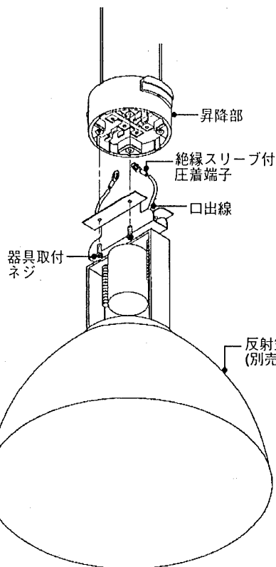
安定器別置タイプ
