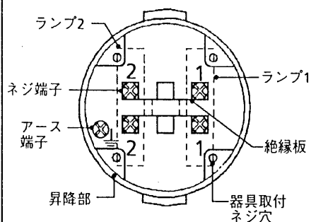
安定器昇降タイプ
