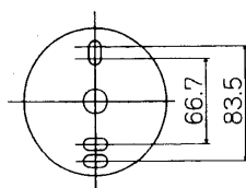
本体取付ピッチ
