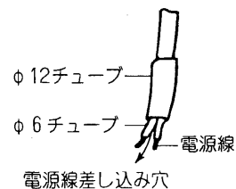
保護チューブの取り付け方
