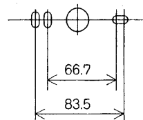
本体取付ピッチ
