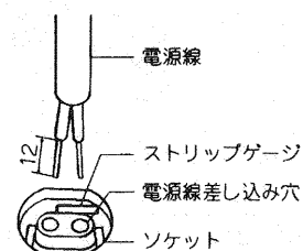
図-2 電源線接続方法
