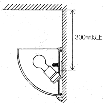
図-1 天井からの取付距離
