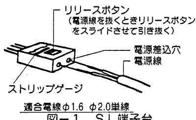
図-1 SL端子台
