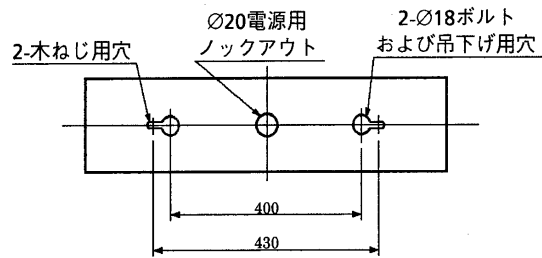
背面仕様図
