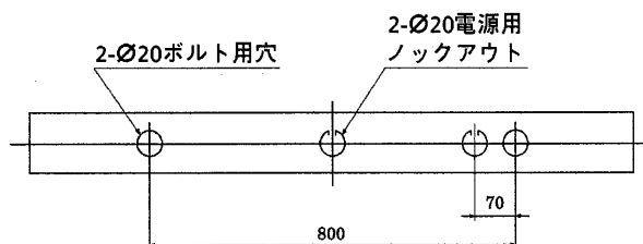
背面仕様図
