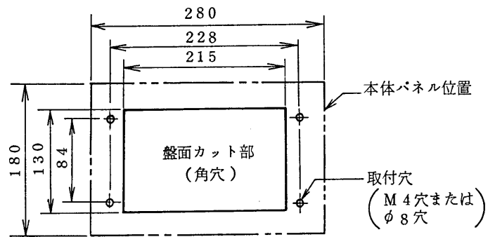
盤面取付穴加工図
